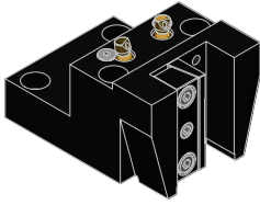
OD TURNING HOLDER .....pg 32
