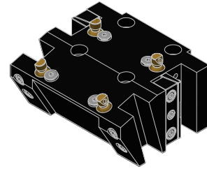
QUAD OFFSET OD TURNING HOLDER .....pg 12
