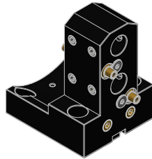
DOUBLE BORING BAR HOLDER .....pg 23
