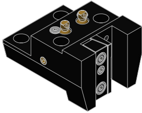
OD TURNING HOLDER .....pg 20
